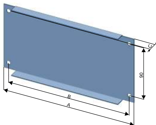
Montážny plech široký pozinkovaný BMS
